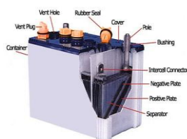
Gambar 2 baterai
